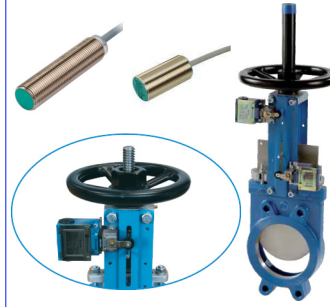
eindschakelaars mechanisch met rolstiftbediening of met naderingsschakelaars PNP NO 3-draads
